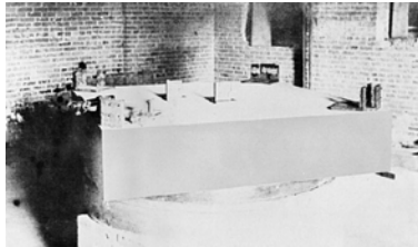
Michelson's & Morley's actual apparatus, the interferometer .
