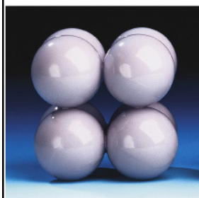
Simple cubic
